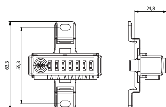
vodorovná montáž
